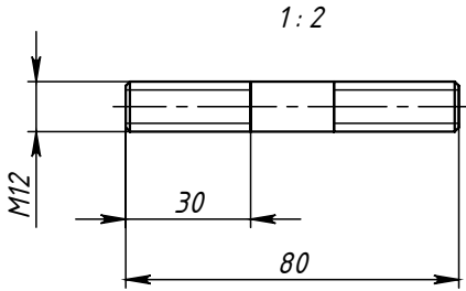
Поз.3 (Шпилька)
