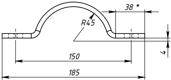
Поз.2 (Полухомут)
